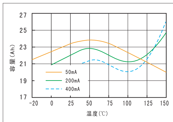
容量与温度关系曲线(2.0V终止)
