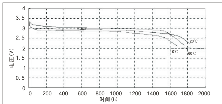
不同温度下放电曲线(47kΩ)
