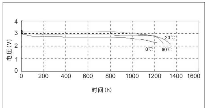
不同温度下放电曲线(15kΩ)
