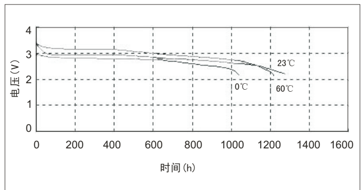
不同温度下放电曲线 (7.5kΩ)
